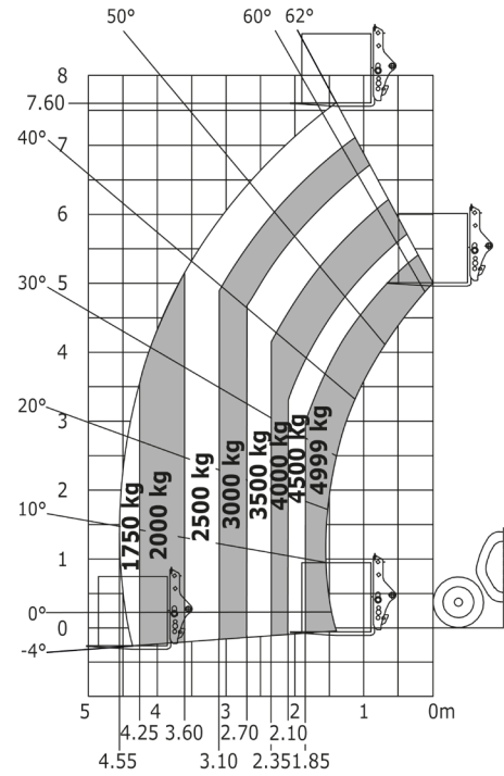
Abaque tout terrain (EN 1459 B) Centre de gravité 500 mm
