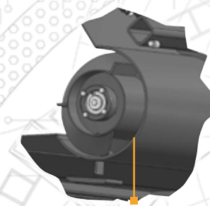
Auge en 8mm sur Omegamax ou auge en 6mm Inox (304L en option)
