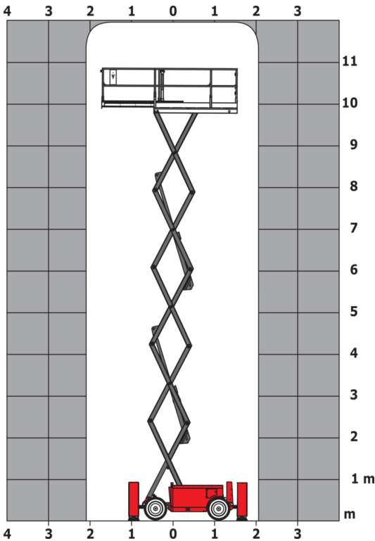
Abaque de charge pour nacelles métrique
